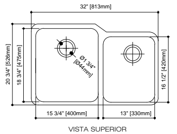
VISTA SUPERIOR
