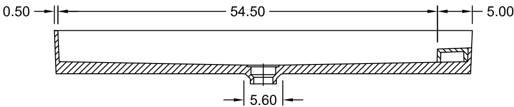
SECTION A-A
