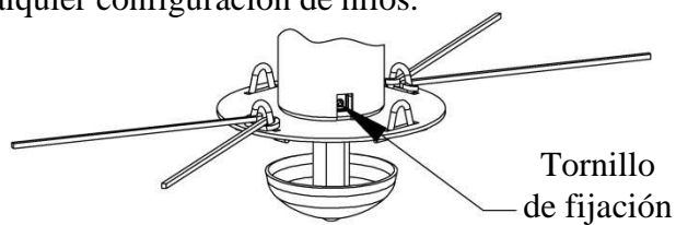
Configuración con 2 hilos Se ilustra ajustada a una altura de corte alta
