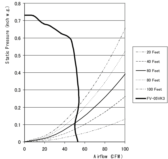
Fan Curve FV-05VK3
