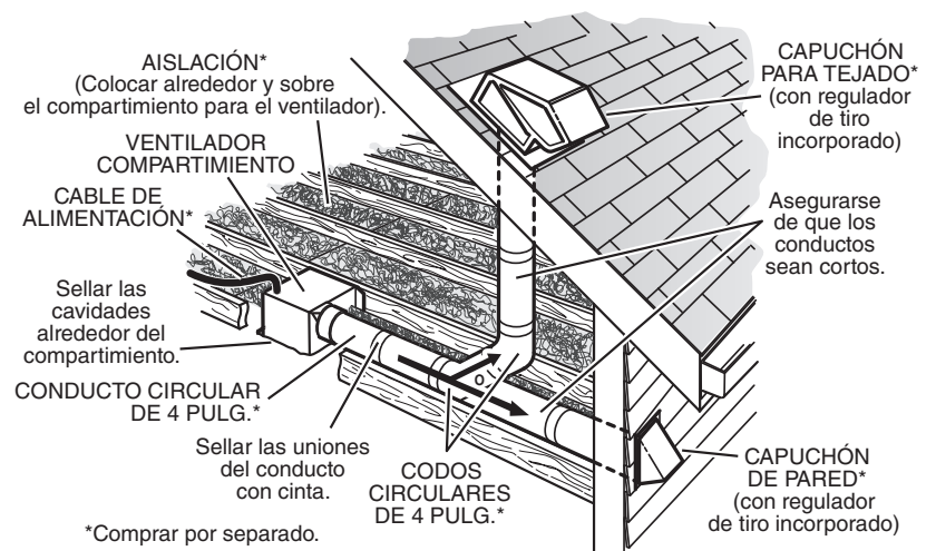
CUBIERTA MONTADA EN UNA VIGUETA "1" Se requiere una estructura adicional para las aletas de montaje. Descarga paralela a las viguetas.
