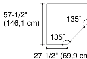
Detalle de la abertura para el estilo de borde de sobreponer
