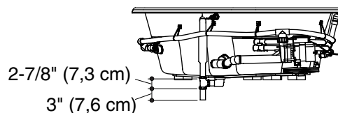
Detalle de la abertura para el estilo de borde de sobreponer
