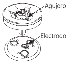
Quemador frontal derecho (en algunos modelos)
