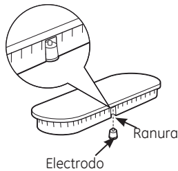
Electrodo Ranura
