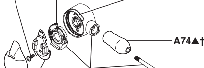
RP32103 Handle Assembly Ensamble de la Manija Poignée
