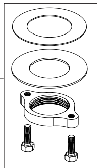
RP101016 Mounting Kit Juego de piezas para la instalación Kit de montage
