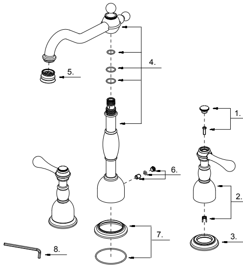
D306957T (VA)
