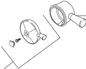
RP49098▲ Temperature Knob, Cover & Screw Perilla de la Temperatura, Cubierta y Tornillo Poignéé de Réglage de Température et Vis
