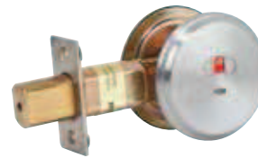
QDB285 Indicator
