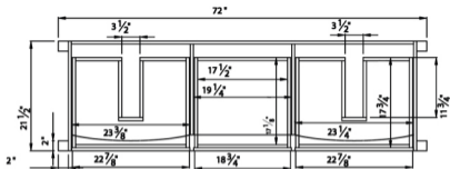
TOP
