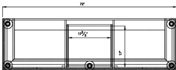
TOP
